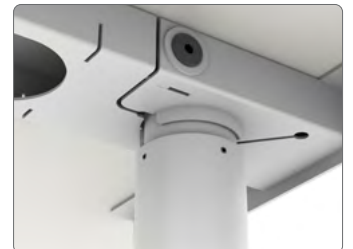
Samling af InLINE, SQUARE og SWITCH søjle med én umbracoskrue
